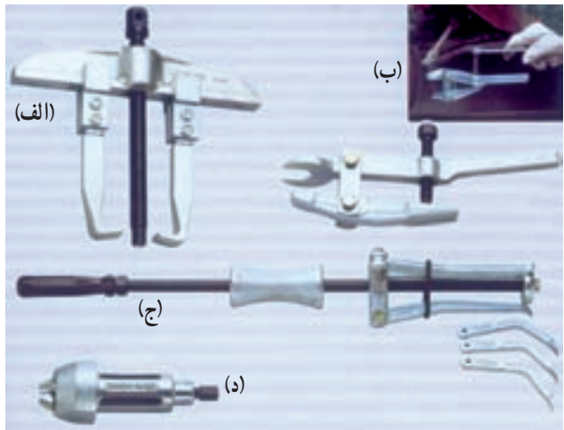
شکل ۱۲-۱- انواع پولی کش‌ها الف- پولی کش با دو بازوی کشویی. ب- پولی کش برای باز کردن پروانه‌های خنک‌کن آلومینیمی و پلاستیکی موتورها. ج- پولی کش ضربه‌ای. د- ابزار خارج‌کننده کُس بلبرینگ
